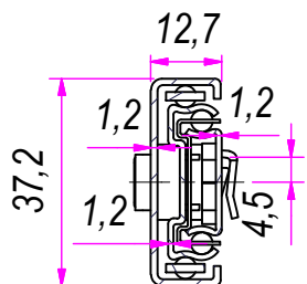
SEZ. A-A
