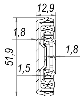
SEZ. A-A
