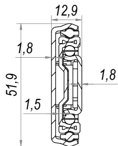
SEZ. A-A
