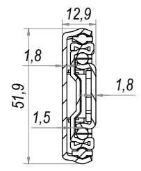
SEZ. A-A
