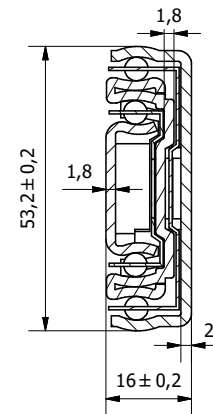
C-C ( 1:1 )
