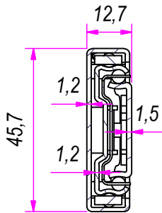
SEZ. A-A
