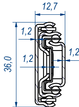
SEZ. A-A
