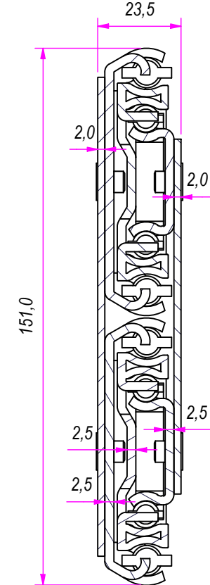
SEZ. A-A
