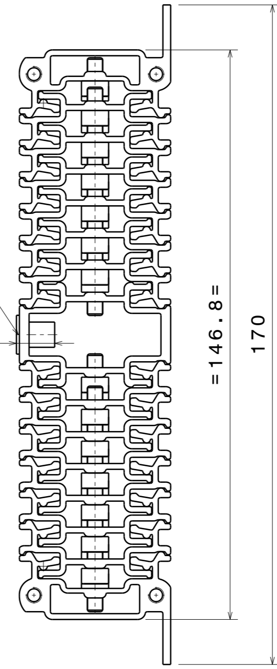
Left view Scale: 1:1
