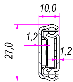
SEZ. A-A
