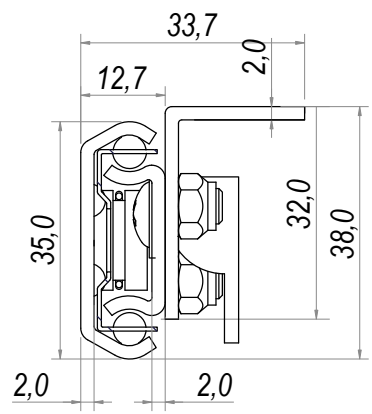
SEZ. A-A
