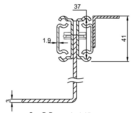
Sez.B-B scala 1:15
