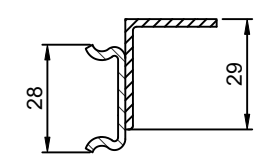
Sez.C-C scala 1:15
