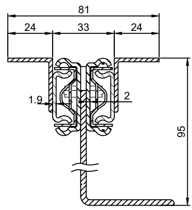
Sez.A-A scala 1:15
