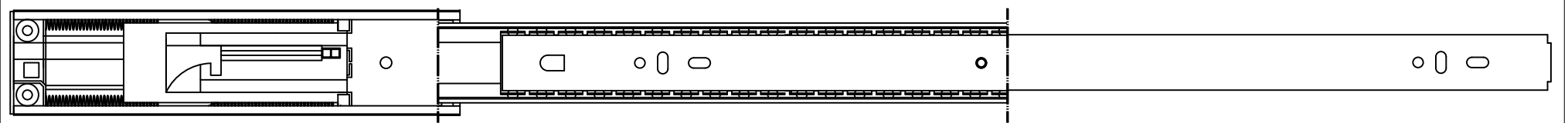
A-A (1.5 : 1)
