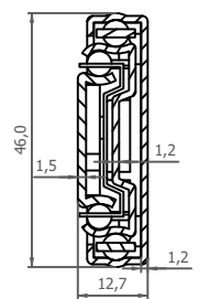
A-A (1.5 : 1)
