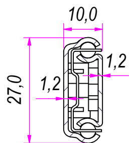
SEZ. A-A
