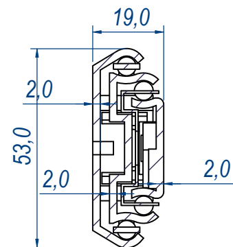
SEZ. A-A
