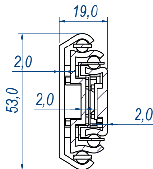
SEZ. A-A
