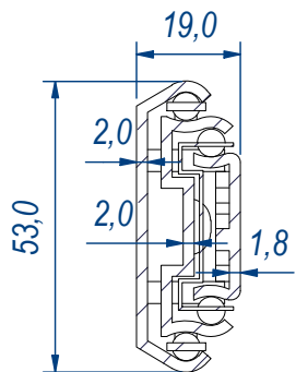
SEZ. A-A
