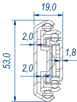
SEZ. A-A
