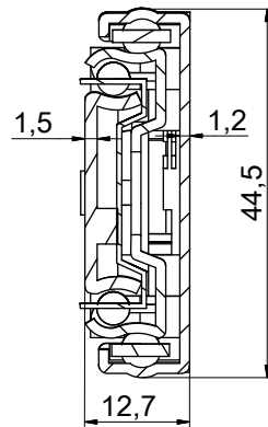
A-A (1:1)
