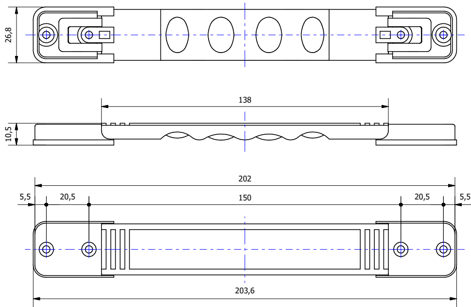
SCALE 1:1,25
