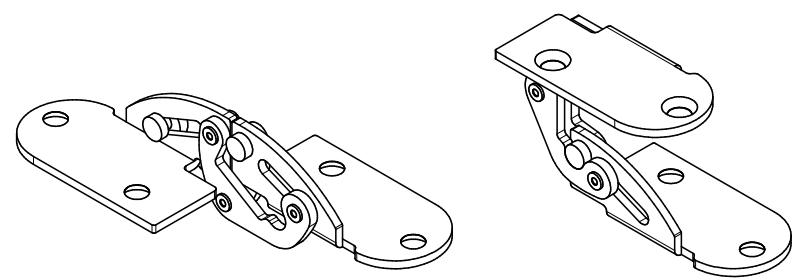
SCALE 1:1
