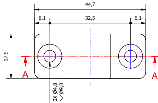
SCALE 1,5:1
