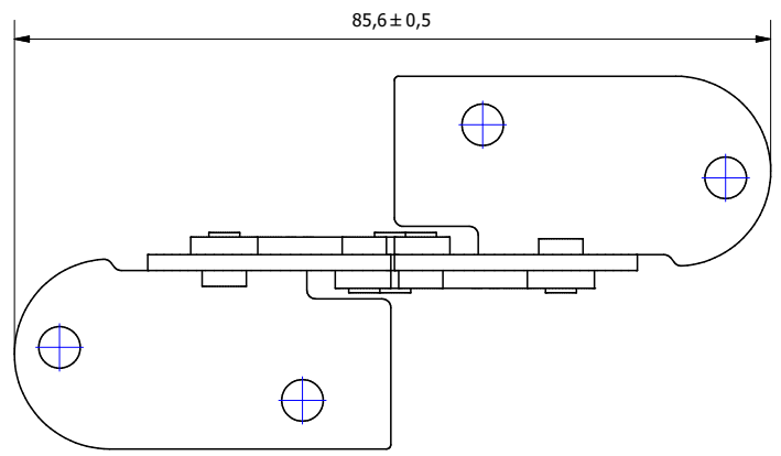
SCALE 1,5:1
