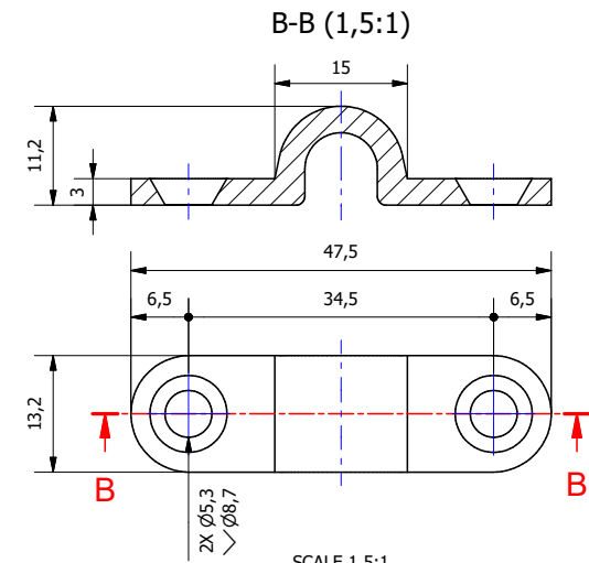
SCALE 1,5:1
