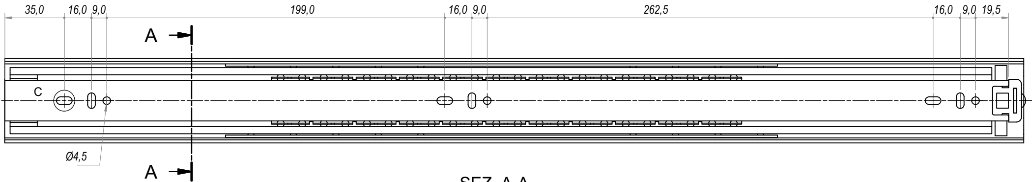
SEZ. A-A
