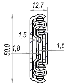
SEZ. A-A
