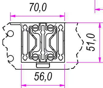
C (1 : 3)
