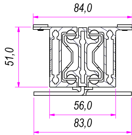
SEZ. A-A
